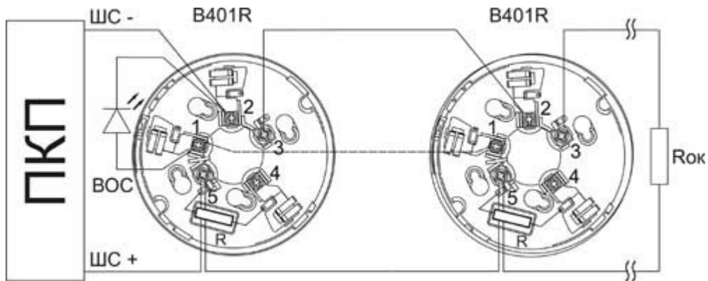
Схема подключения баз В401R, В401R-1000 к двухпороговому ПКП (с распознаванием одного и двух сработавших извещателей в шлейфе)
